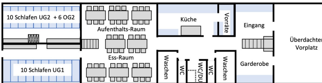
PHD Erdgeschoss
